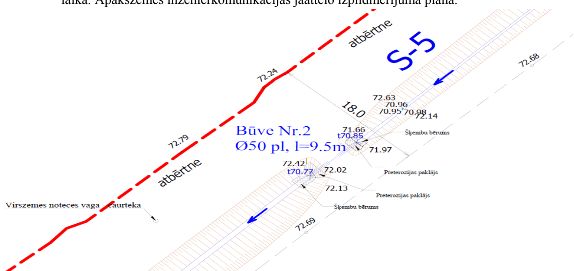
2.attēls. Izpildmērījumā piemērs ar uzmērītu grāvja trases platumu, grāvi, attēlotu grāvja numuru, atbērtni, caurteku, nostiprinājuma veidu un virszemes noteces vagas veidu.
