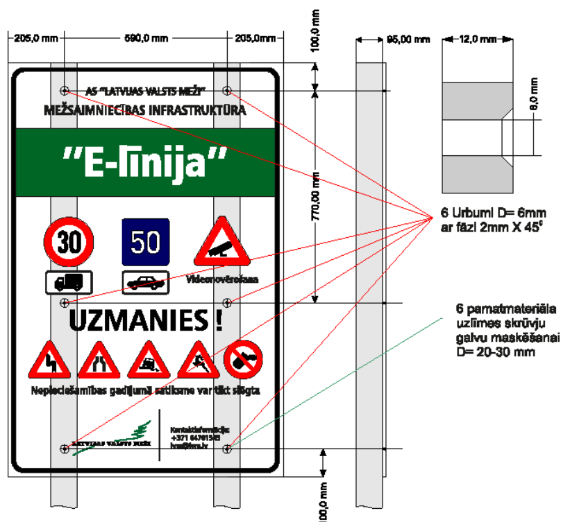
1.att. Skrūvju izvietojuma shēma.
