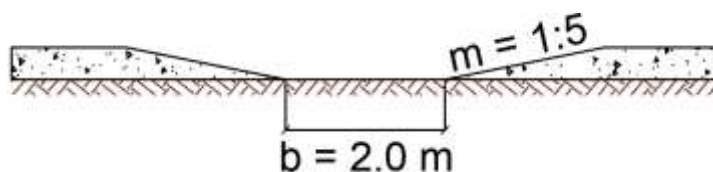
2. attēls. Noteces vagas šķērsriezums paralēli grāvja asij
