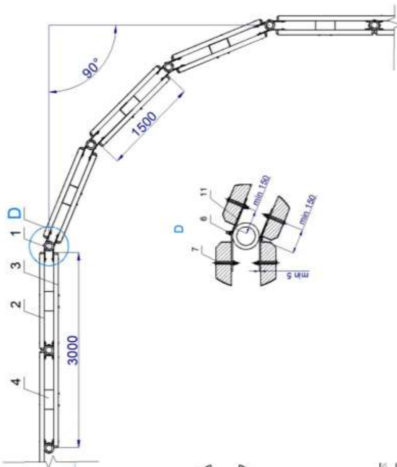
Koka atvairbarjeras pagrieziņa detalizācija
