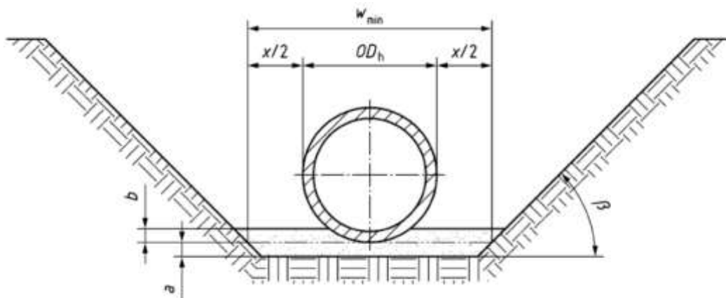
1. attēls. Minimālais tranšejas platums
