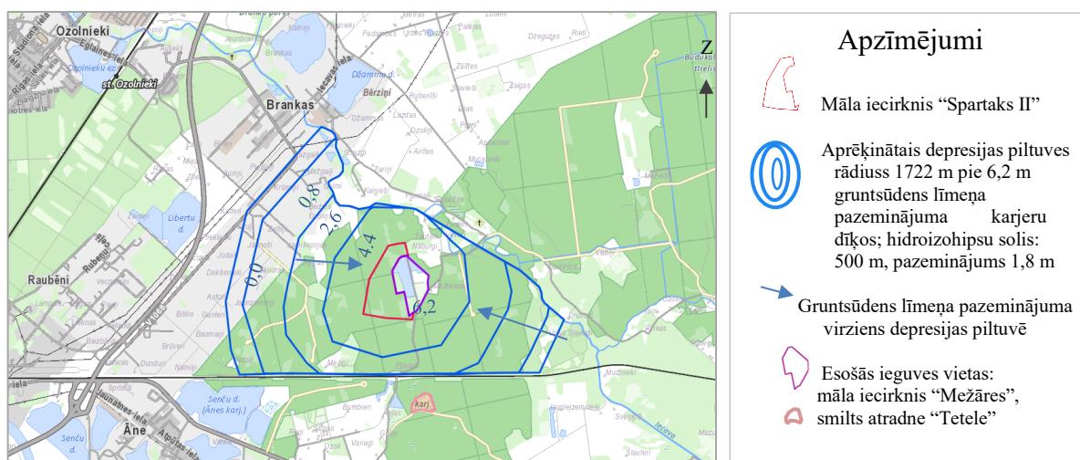
3.46.att. Aprēķinātā summārā depresijas piltuve atradnes “Spartaks III” iecirknim “Spartaks II” un “Mežāres”, M 1:30000
