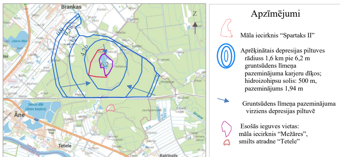
3.44.att. Aprēķinātās depresijas piltuves rādīss ap iecirkņa “Mežezers” teritoriju, M 1:30000
