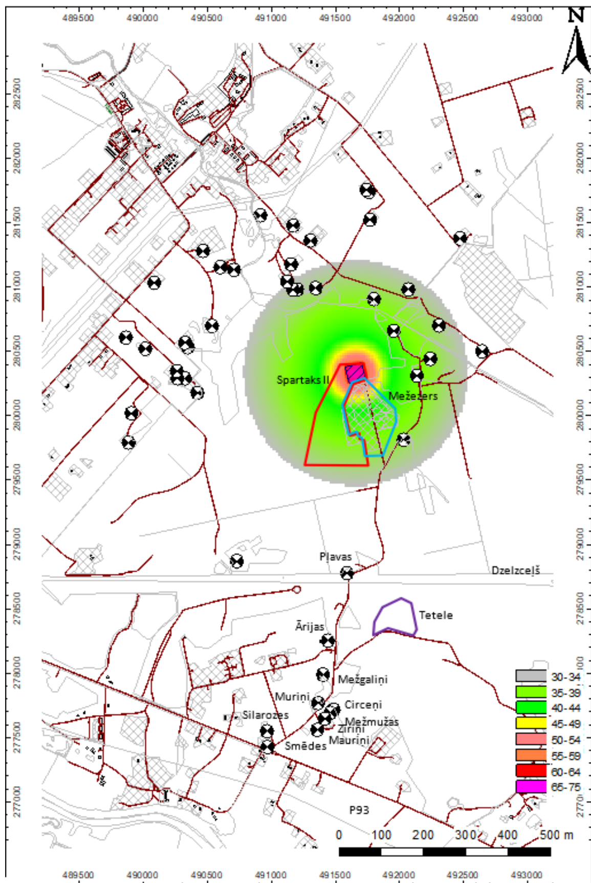
3.27. att. Aprēķinātais iecirkņa “Spartaks II” trokšņa līmenis tikai no ražošanas (no 1 ieguves laukuma) L_{\text{dienā}} .
